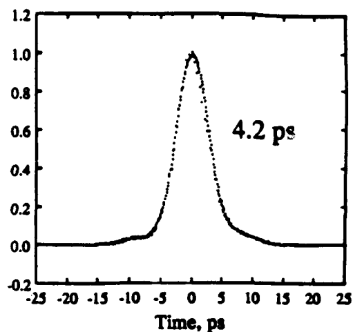
Fig. 2: RPM Nd:YLF autocorrelation
