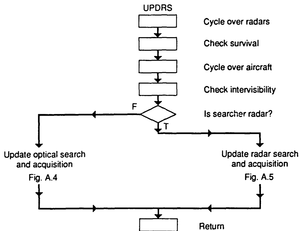
Fig. A.5—Update searchers (UPDRS) flow chart
