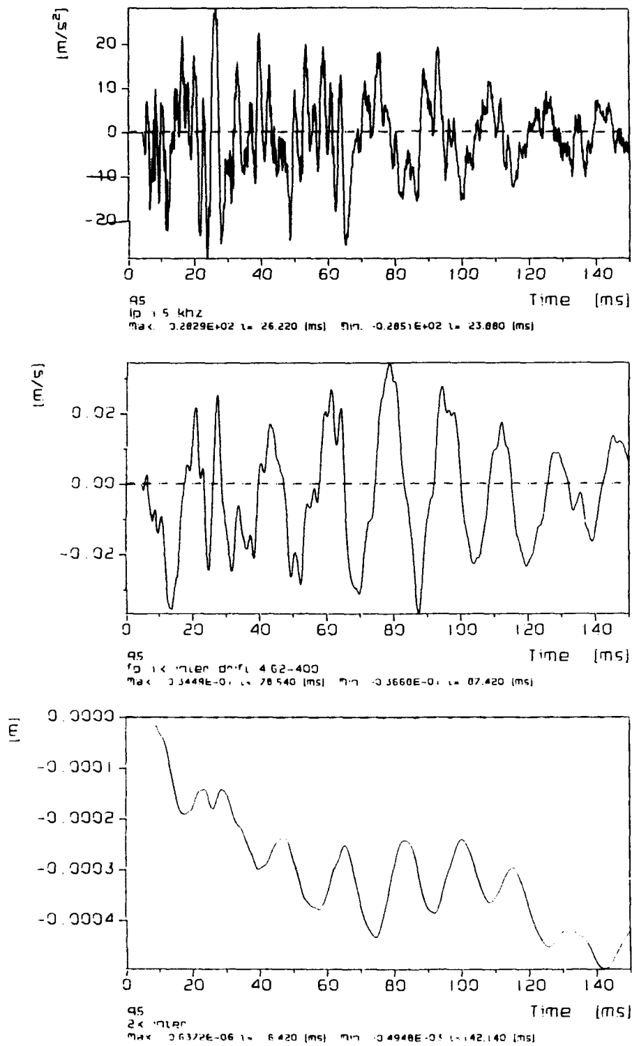
Figure 33 Accelerometer A5
