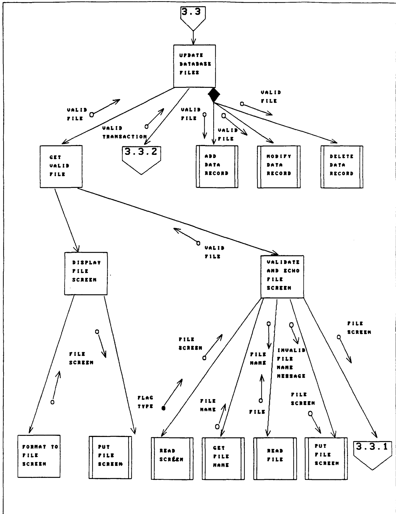
Fig. D-10, UPDATE DATABASE FILES.
