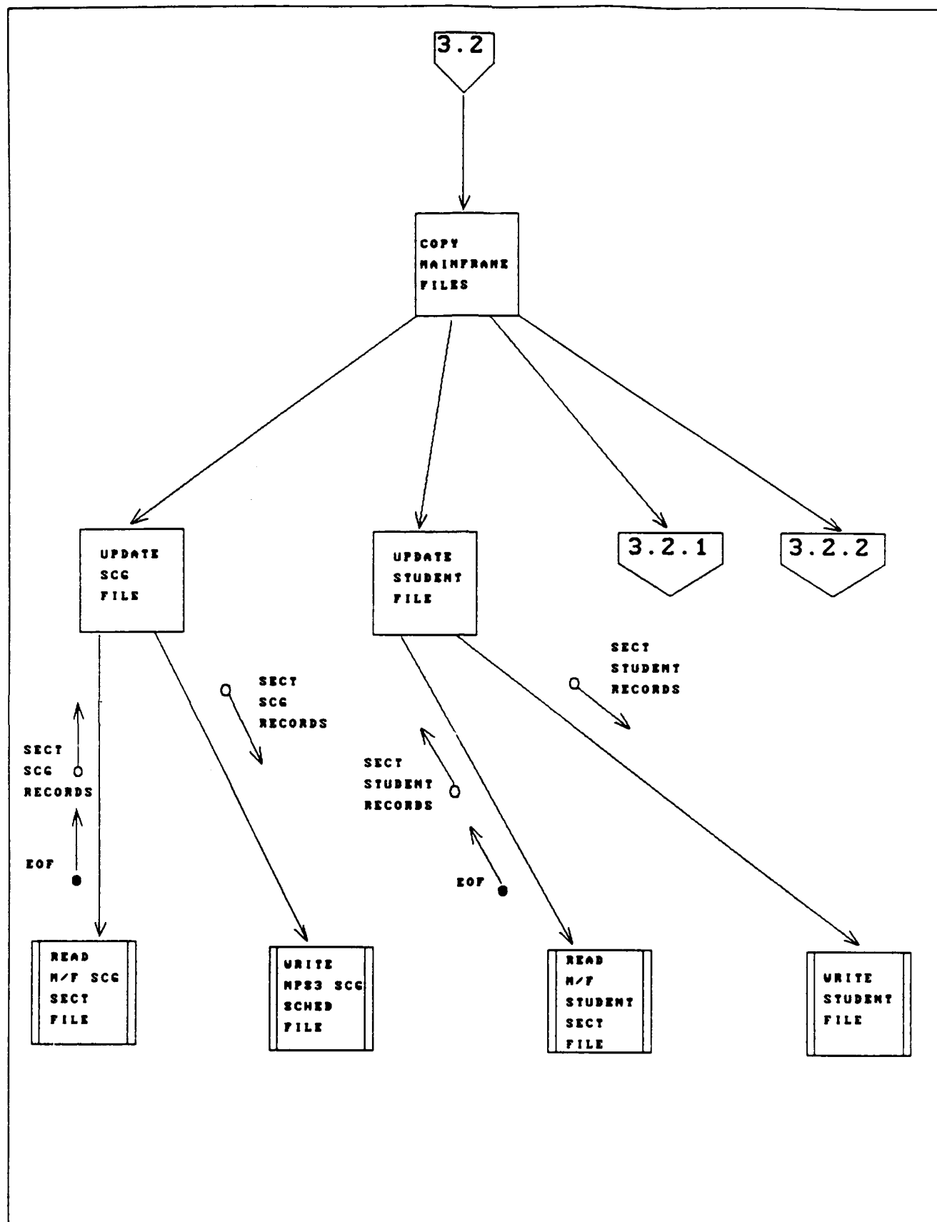
Fig. D-7, COPY MAINFRAME FILES.
