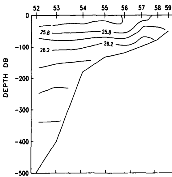
B SIGMA-T
