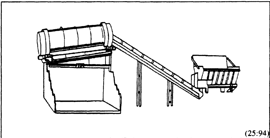
Figure 22. Trommel Screen
