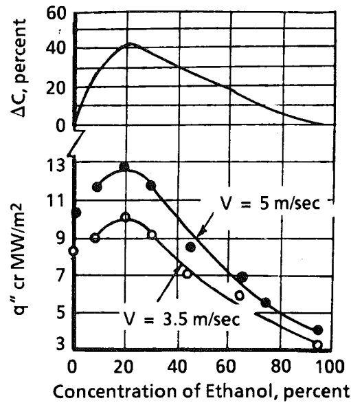
a. Ethanol-water
