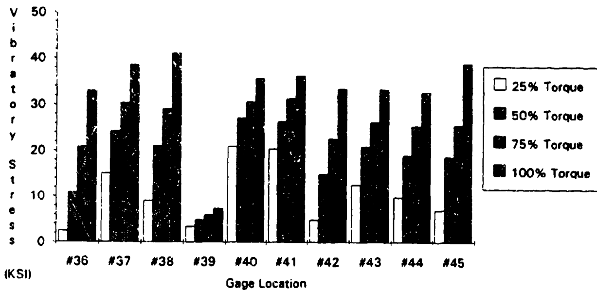
Figure 134. Vibratory Stress, DH Gear Meshing w Lower DH Pinion
