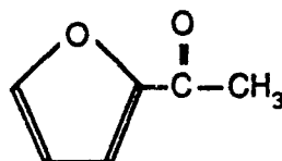
2-Acetylfuran
