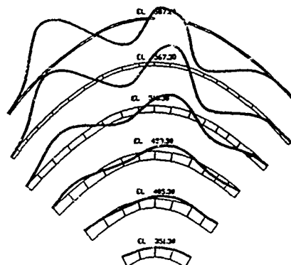
MODE-4 3.68 HZ
