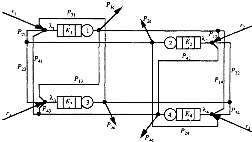
Fig. 8 — A four-queue network
