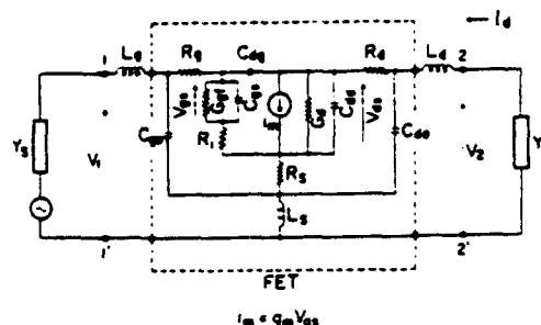
Fig. 1. FET equivalent circuit.
