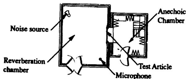
Figure 5. NEL Acoustic TL Test
