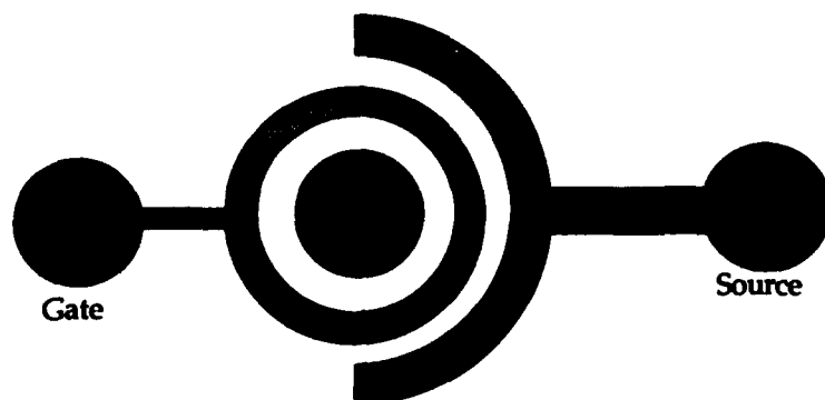
MESFET Structure
