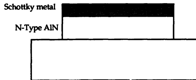
Schottky Diode Mesa
