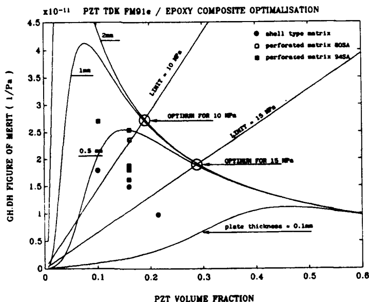
FIGURE 7 1.3.1 piezocomposite optimisation
