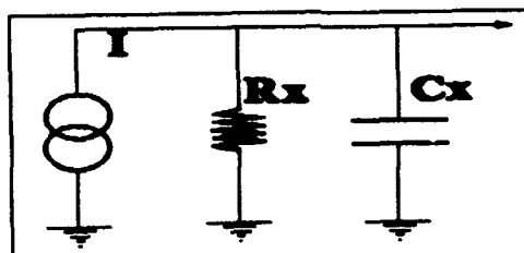
Fig. 1.- Equivalent circuit
