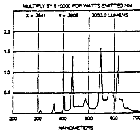
(d) Lite White Deluxe (LWX)
