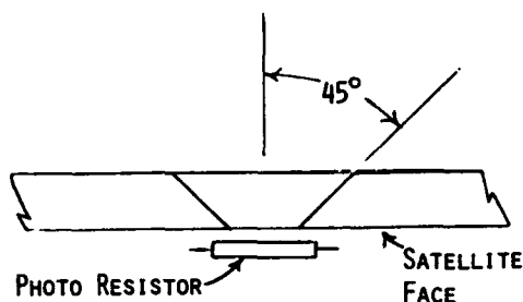
Fig. 1. Light Sensor
