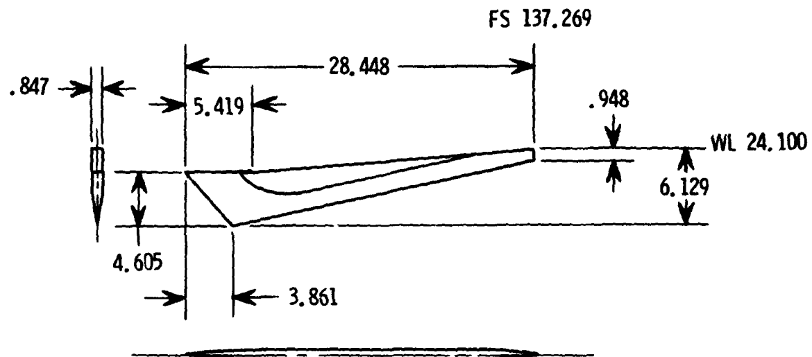
(d) Ventral fin.
