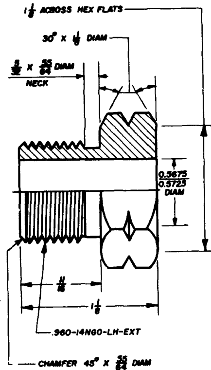
HEX NUT NO. 594
