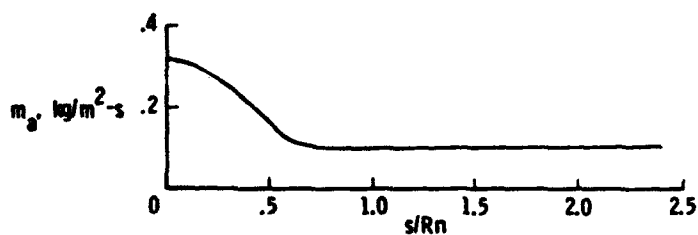
(d) ABLATION RATE DISTRIBUTION
