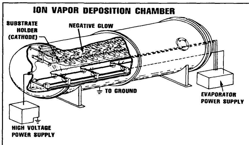
Ion vapor deposition chamber.
