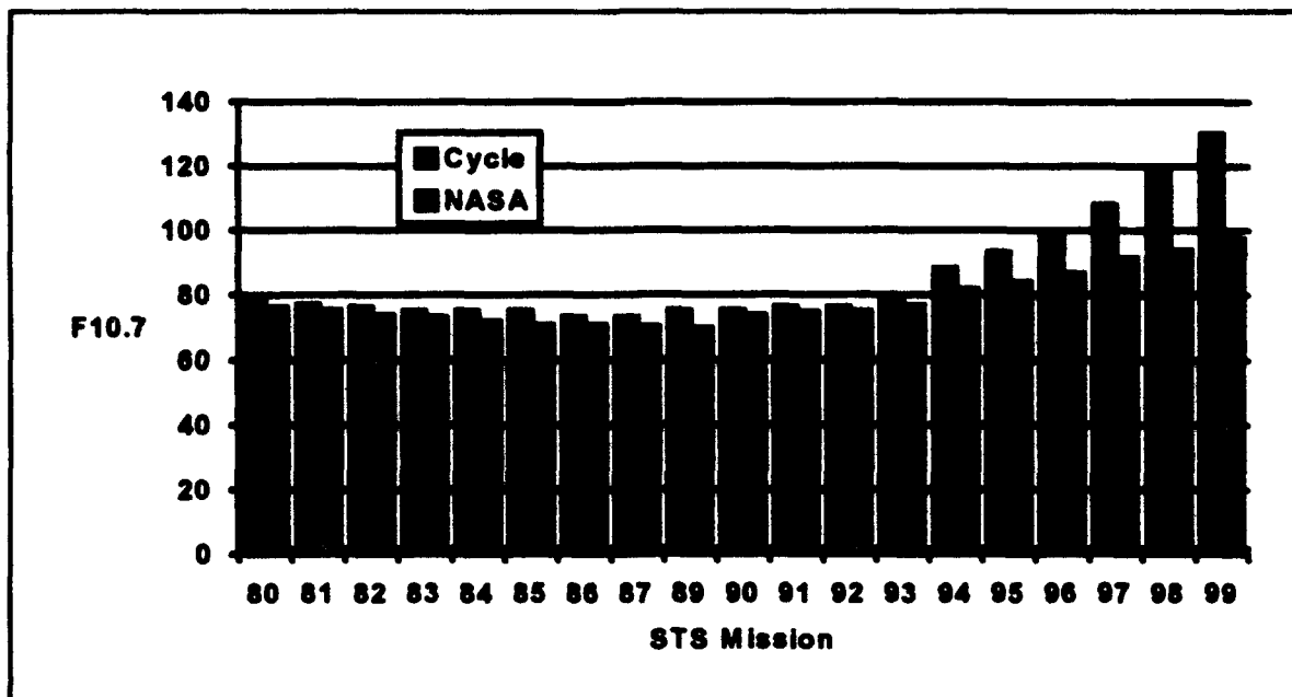
Figure 19. NASA F10.7 Values vs. Predicted Values
