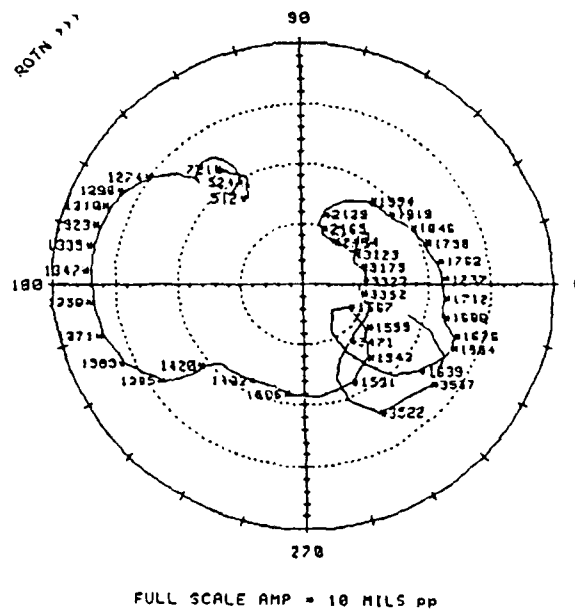
FIG 5 1X POLAR PLOTS
