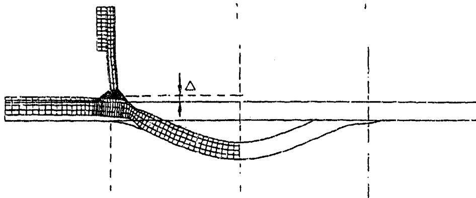
(d) Specimen HY-130 WE3-2, V_0 \approx 230 m/s
