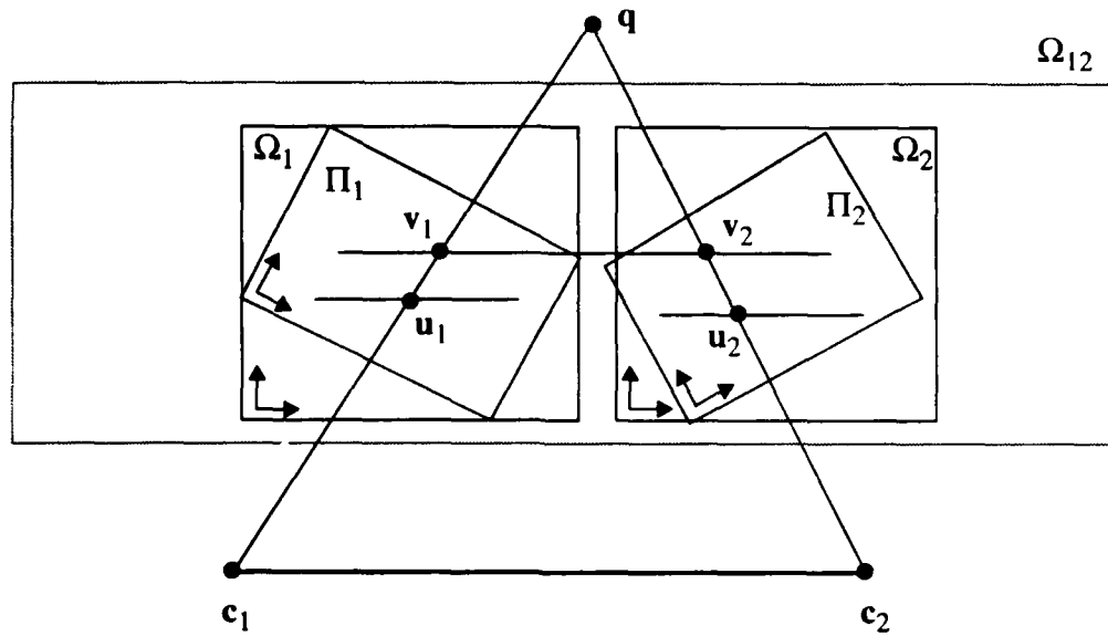
Fig. 8 Image rectification
