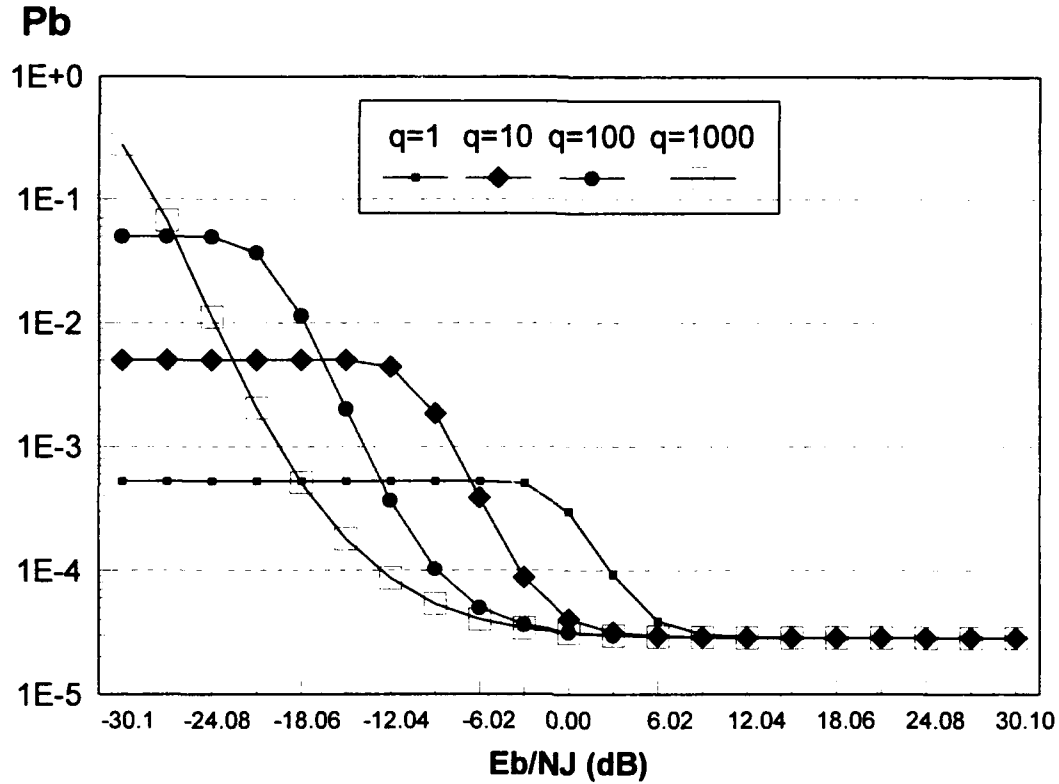
Figure 25. E_b/N_o=13.35\text{dB} , R_b=100 , R_j=100
