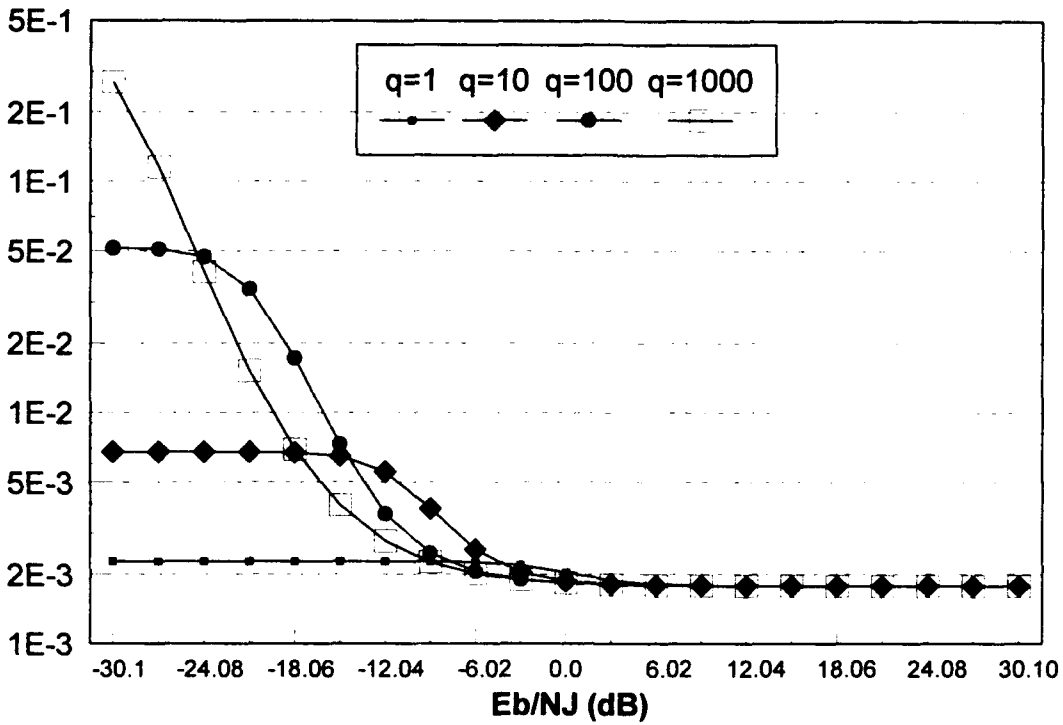
Figure 28. E_v/N_o=13.35\text{dB} , R_b=10 , R_j=10
