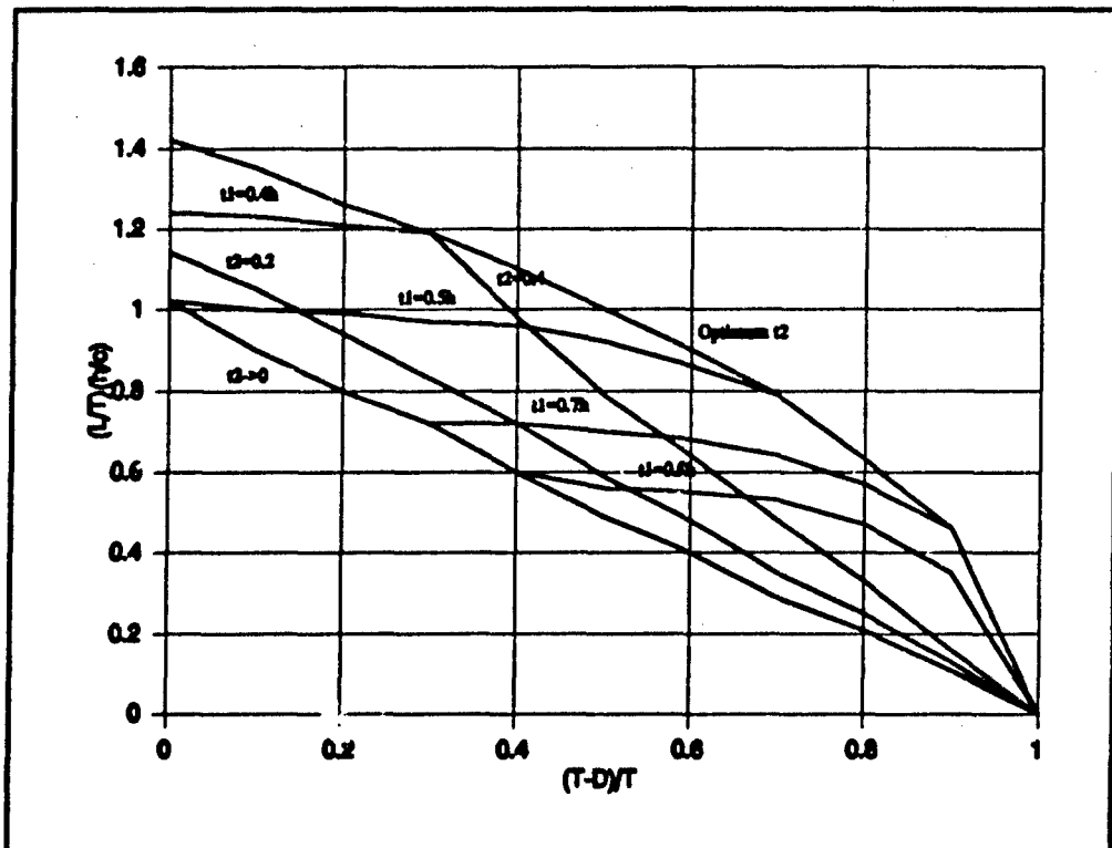
Figure 6: PAR Performance Map
