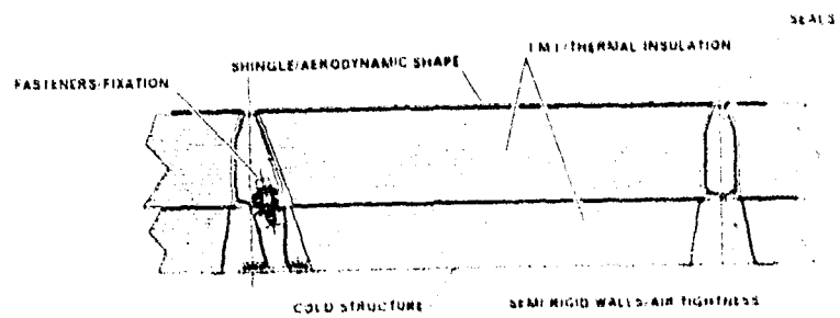
Tuiles extrados
