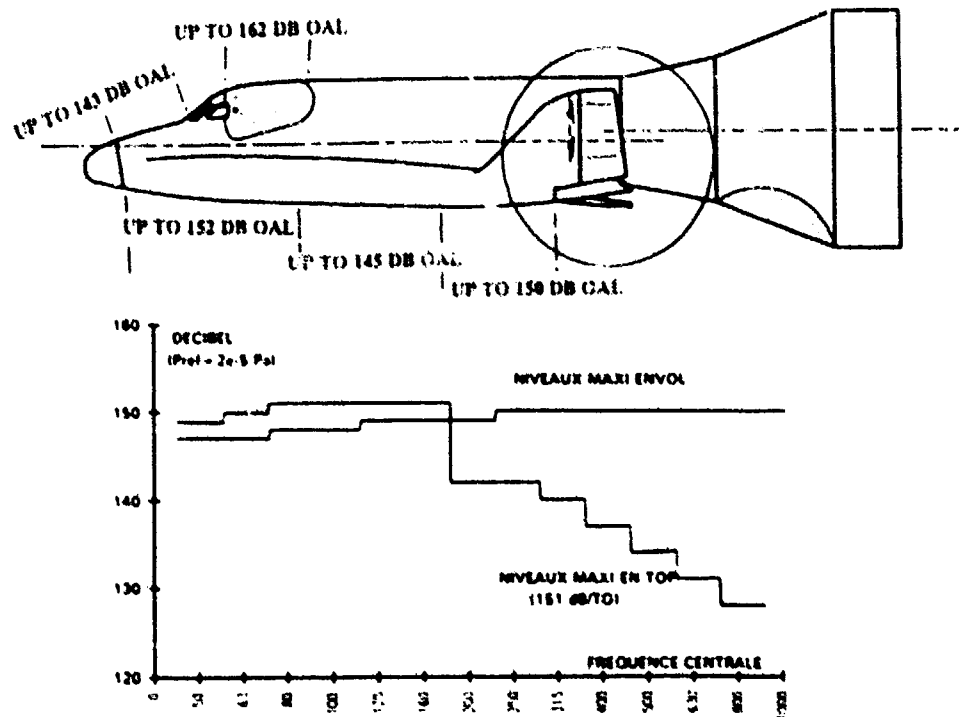
Planche 2 Niveaux de bruit aérodynamique maximum
