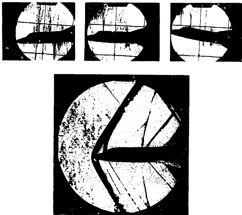
Visualisation strioscopique en supersonique
