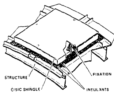
Tuile extrados
