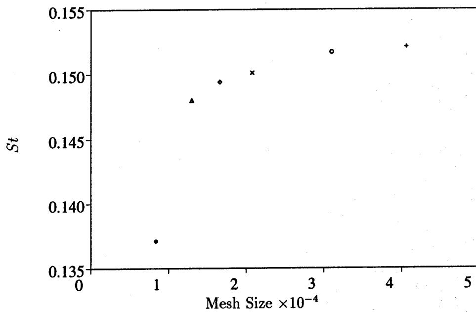
Figure 94: Re=80 ; Strouhal frequency convergence • : 129 \times 65 ; \triangle : 200 \times 65 ; \diamond : 256 \times 65 \times : 320 \times 65 ; \circ : 320 \times 97 ; + : 320 \times 127
