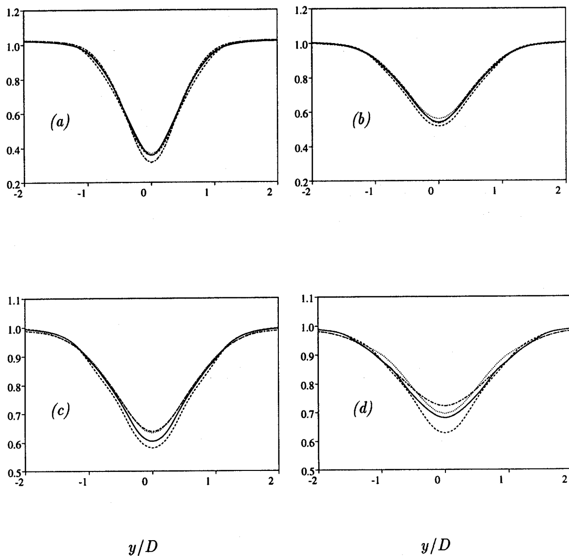
Figure 112: Streamwise velocity \bar{u}/U_\infty at x/D = 2.50 (a), 3.06 (b), 3.54 (c), 4.50 (d) - · - : 88 \times 90 \times 32 ; \cdots : 88 \times 90 \times 48 ; - - - : 116 \times 136 \times 48 — : 174 \times 128 \times 48
