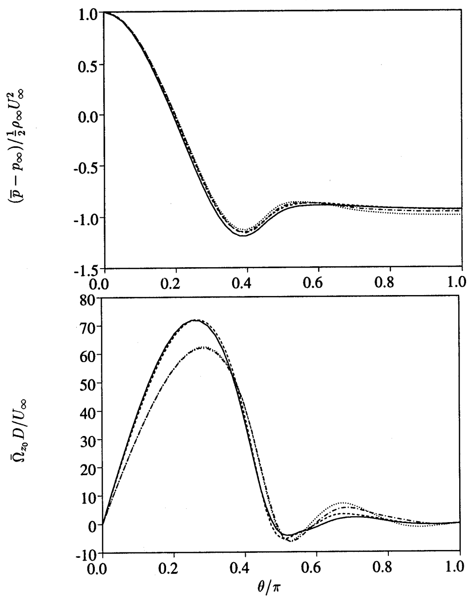
Figure 108: Wall pressure and vorticity - - - : 88 \times 90 \times 32 ; \cdots : 88 \times 90 \times 48 - . - : 116 \times 136 \times 48 ; — : 174 \times 128 \times 48
