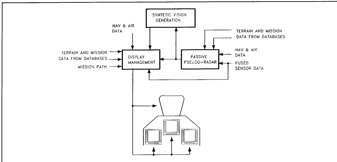
Fig. 5 - Display Area
