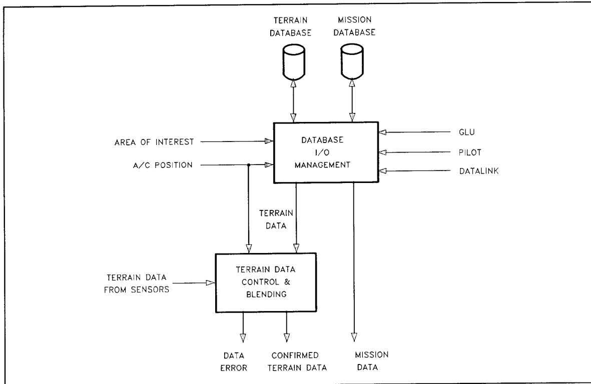
Fig. 3 - Database Area
