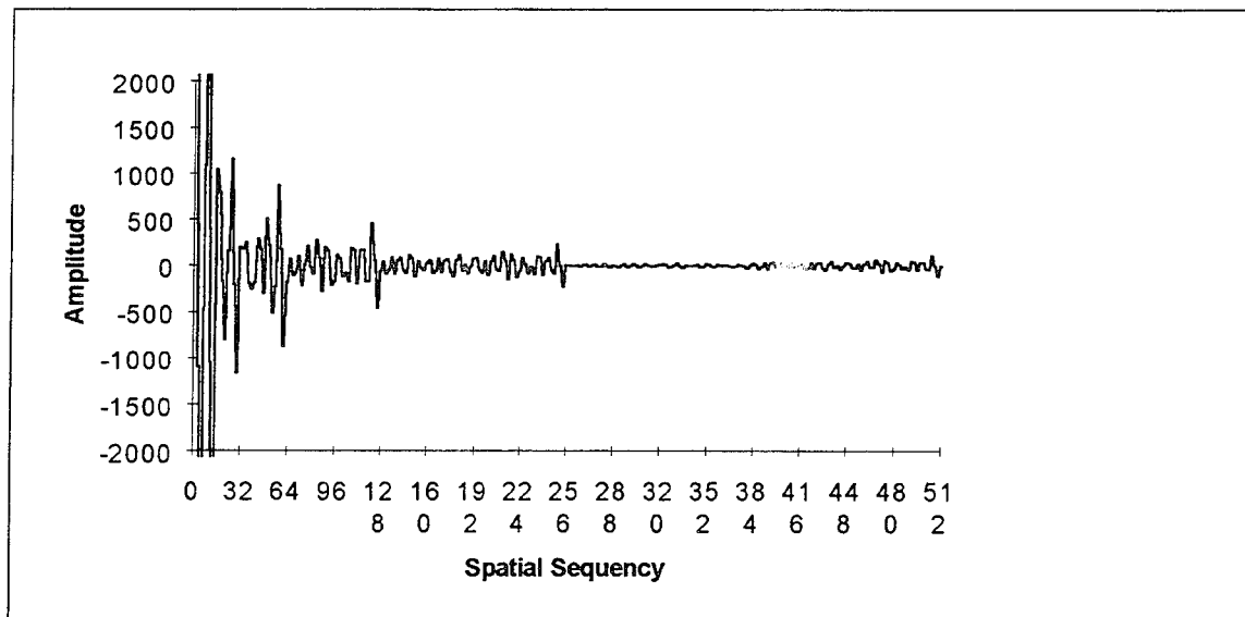
Fig. D-183. Walsh transform of Fig. D-182
