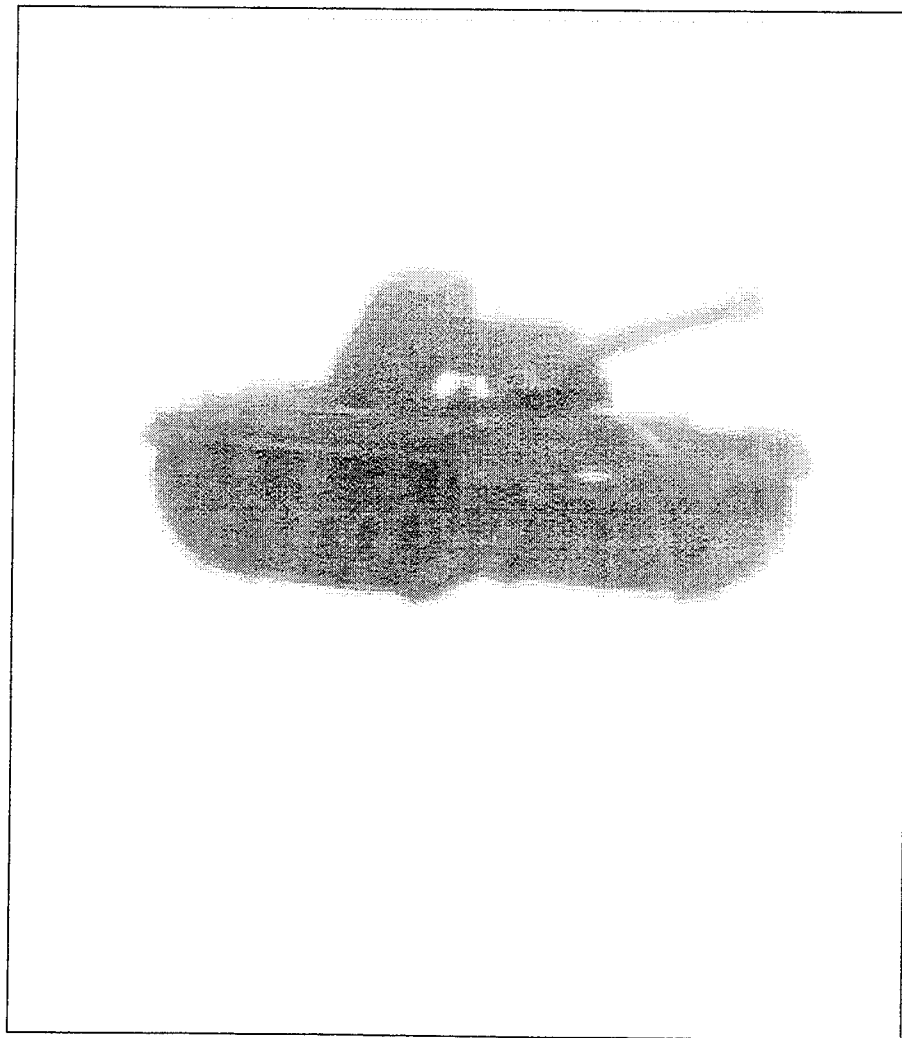
Fig. D-52. T5
