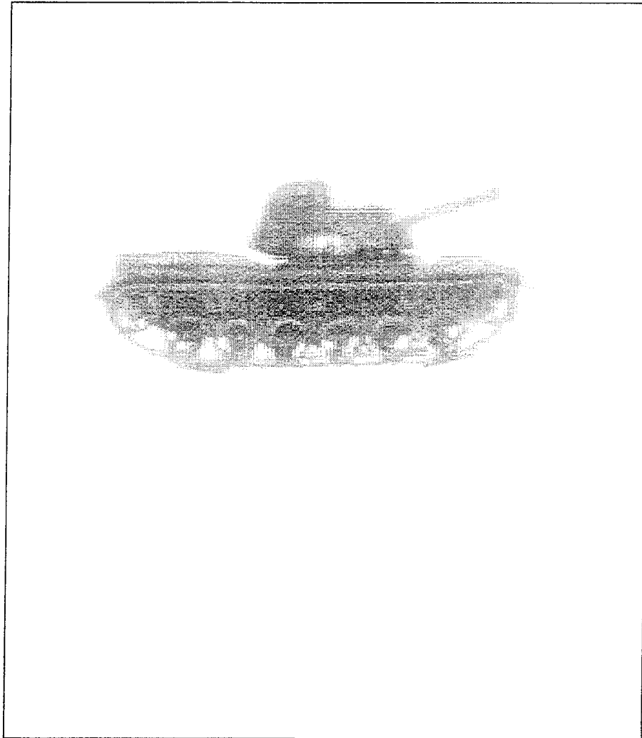
Fig. D-103. T8
