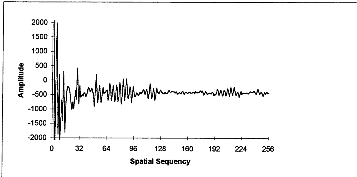
Fig. B-9. Walsh transform of Fig. B-8
