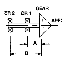
SPIRAL BEVEL
