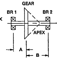
SPIRAL BEVEL
