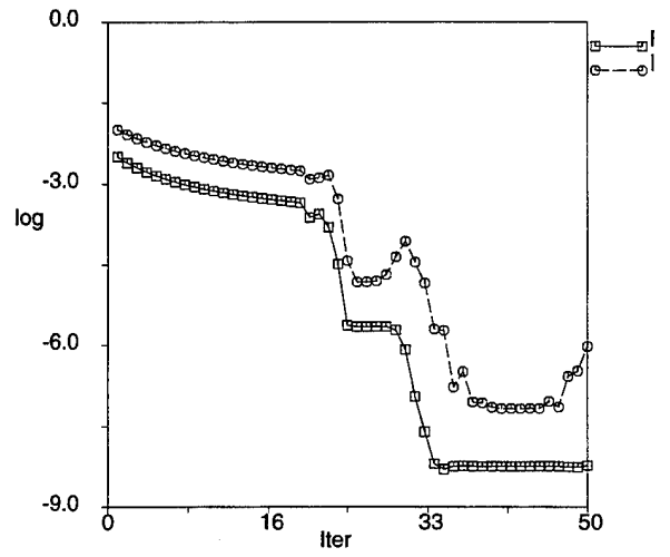
(d) BFGS2.
