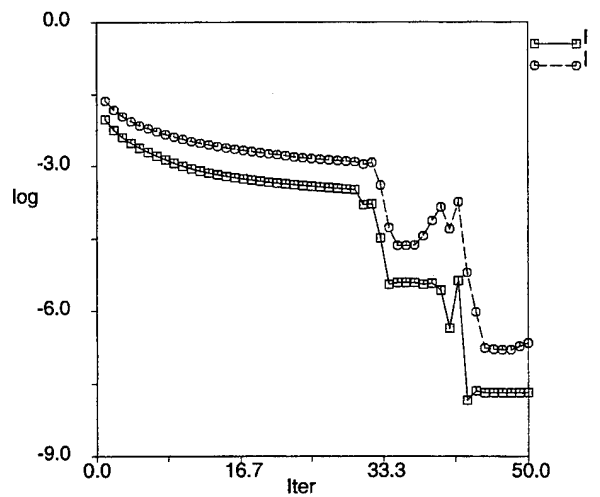
(e) BFGS2.
