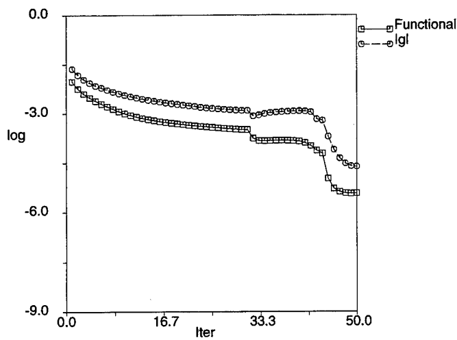
(d) BFGS1.
