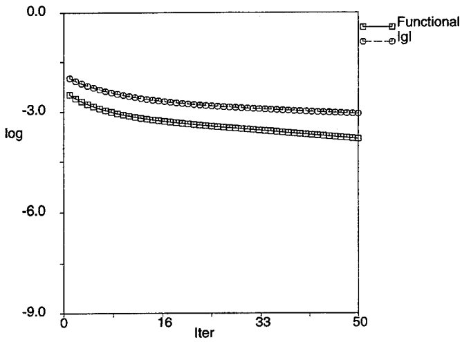
(a) SD1.
