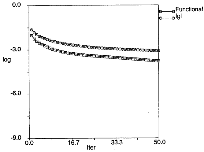
(b) SD1.
