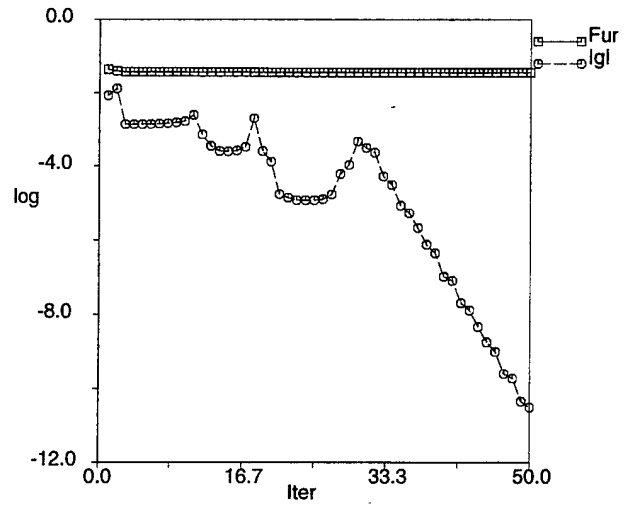
(b) BFGS2.
