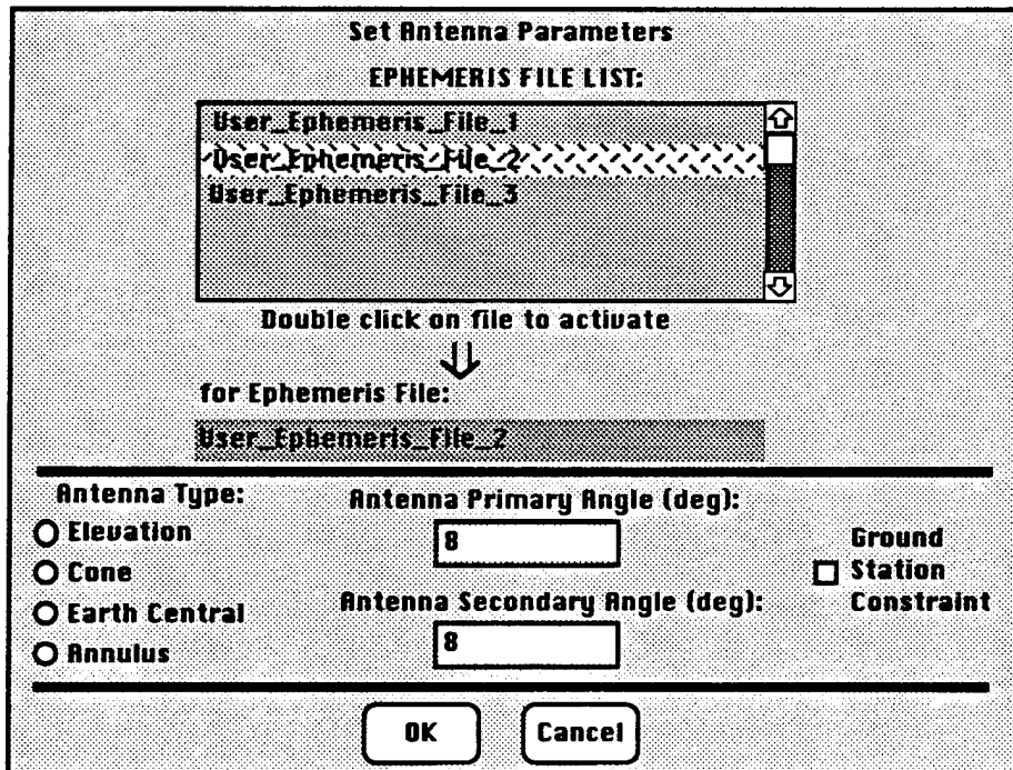
Figure 8-3. Antenna Parameters Dialog
