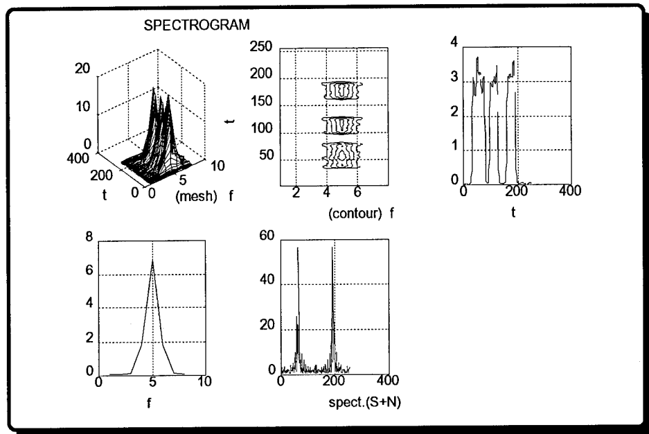
Figure 5.63: OOK Spectrogram (SNR= +20 dB)
