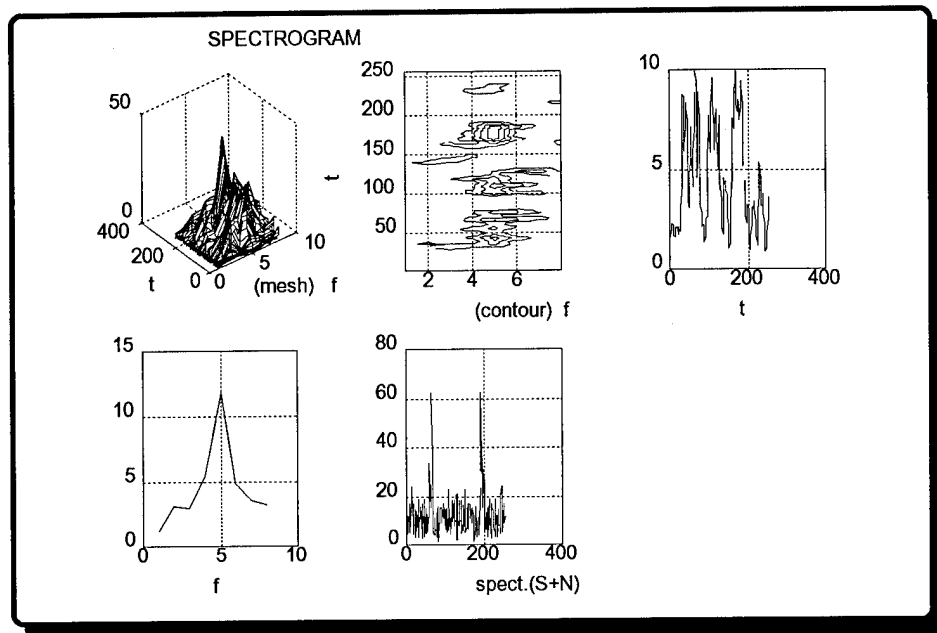
Figure 5.67: OOK Spectrogram (SNR= 0 dB)
