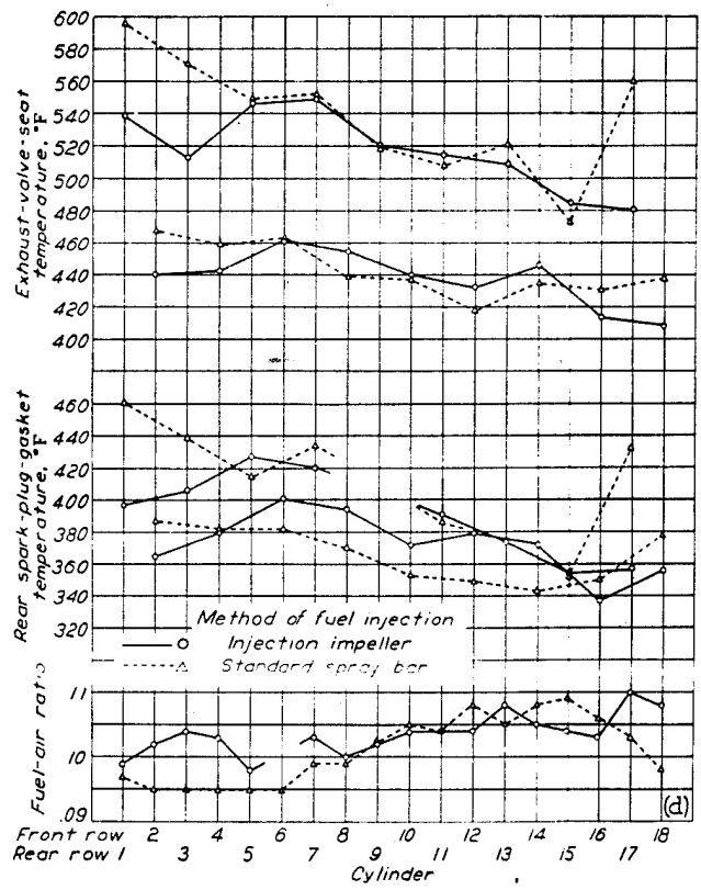
(d) Brake horsepower, 2000; engine speed, 2100 rpm.
