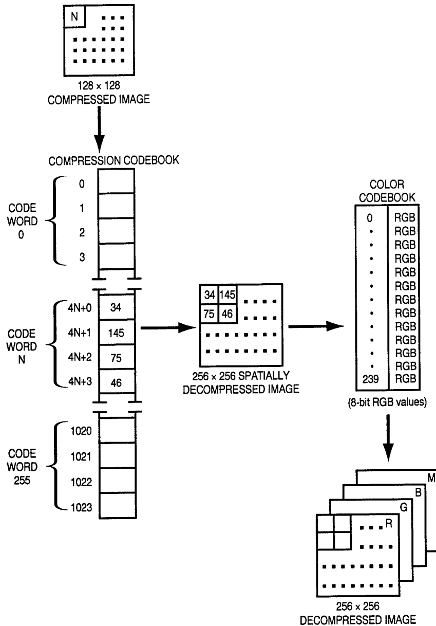
Fig. 4 — CAC decompression
