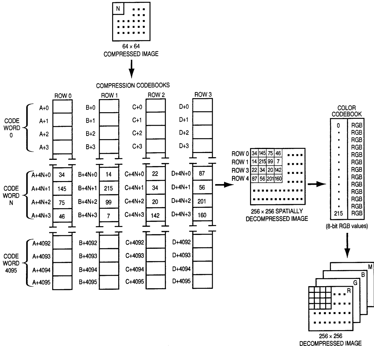
Fig. 5 — CADRG decompression
