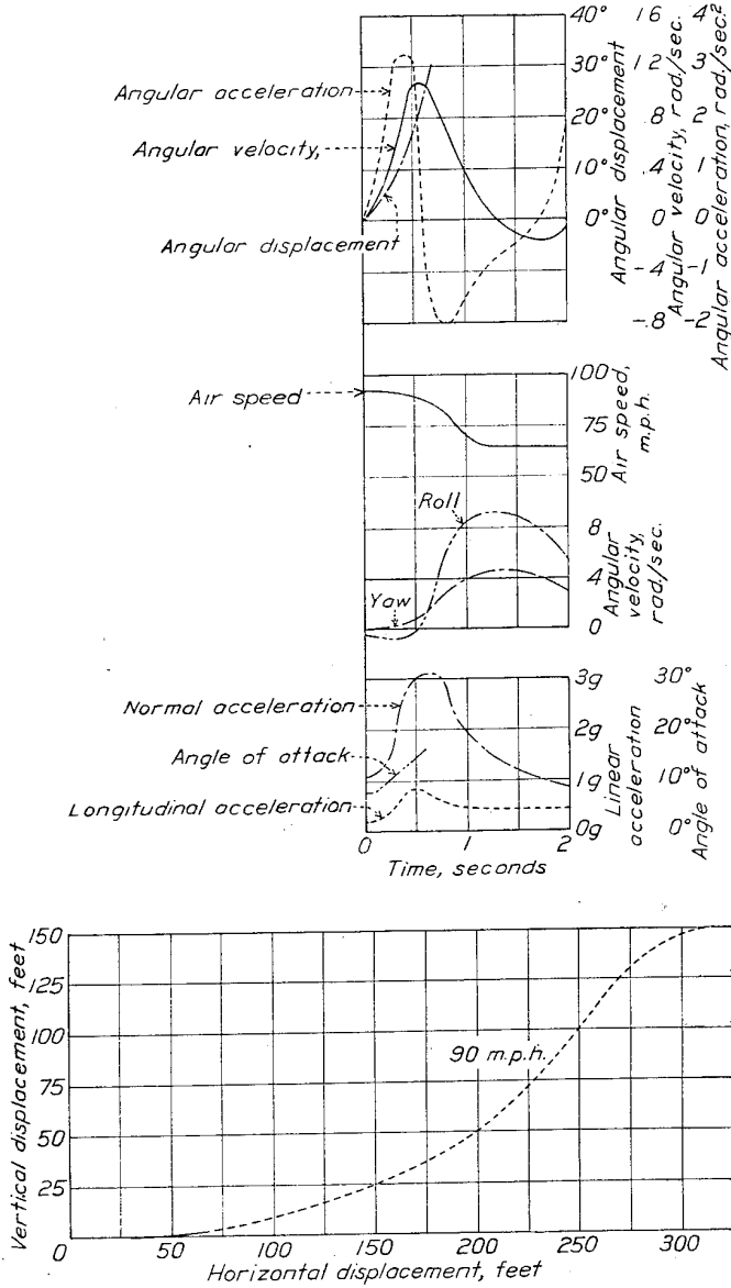
FIGURE 14.—90 m. p. h. abrupt pull-up maneuver
