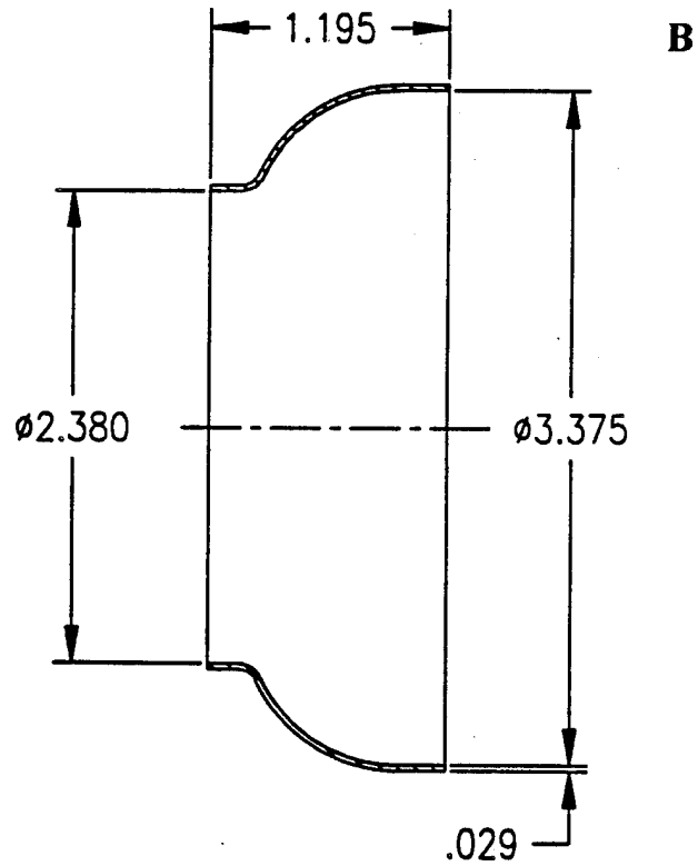
CORONA SHIELD 372657 304L SST
