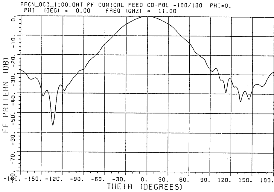
(a) H-plane
