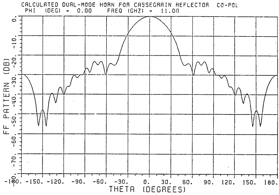
(a) H-plane
