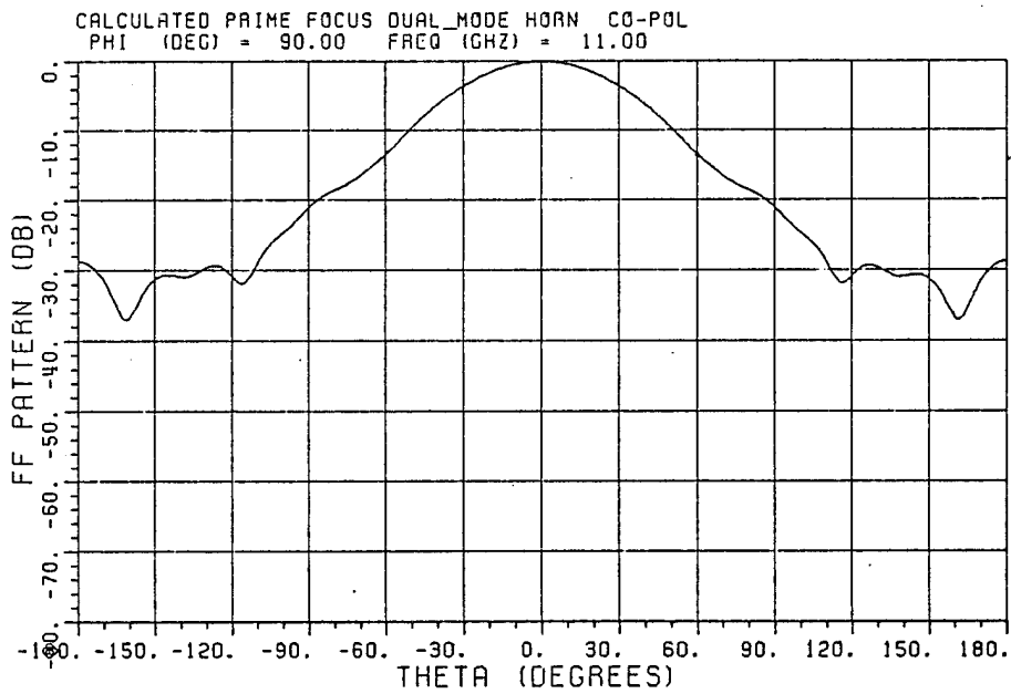
(b) E-plane
