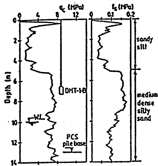
a. DMT-results at Oudenaarde
