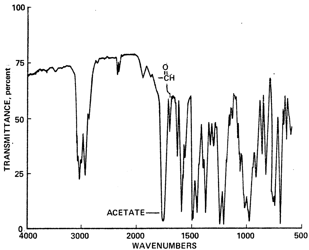
FIG. 3 IR SPECTRUM OF VST
