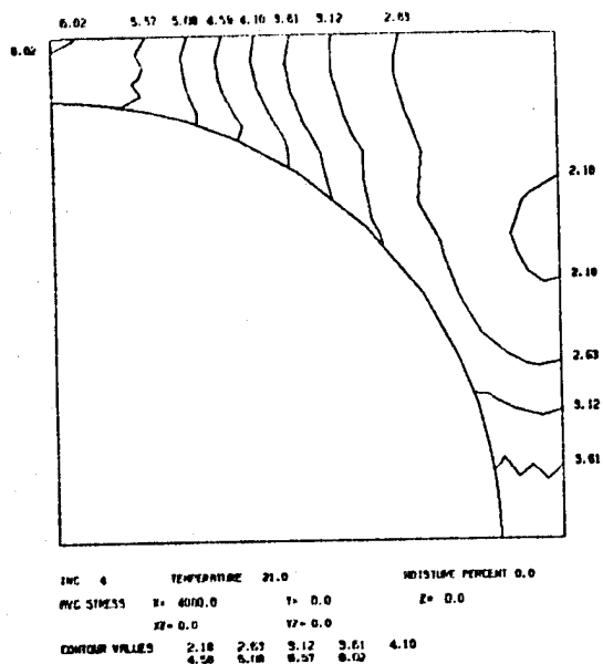
a) Octetedral Shear Stress (ksi)
