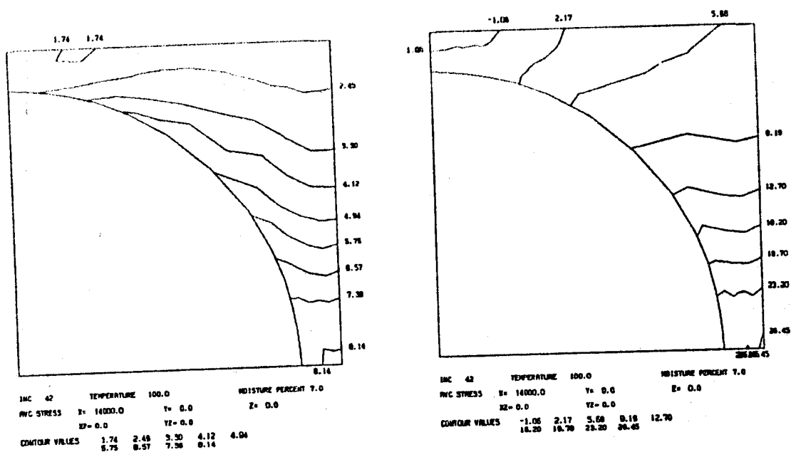
a) Octahedral Shear Stress (ksi) b) Maximum Principal Stress (ksi)
