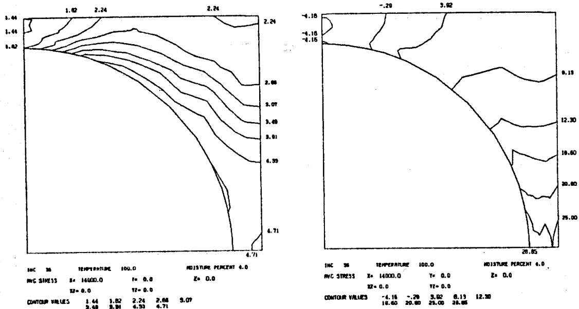
b) Maximum Principal Stress (ksi)
