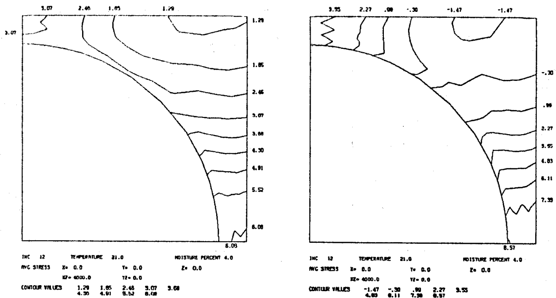
a) Octahedral Shear Stress (ksi)
