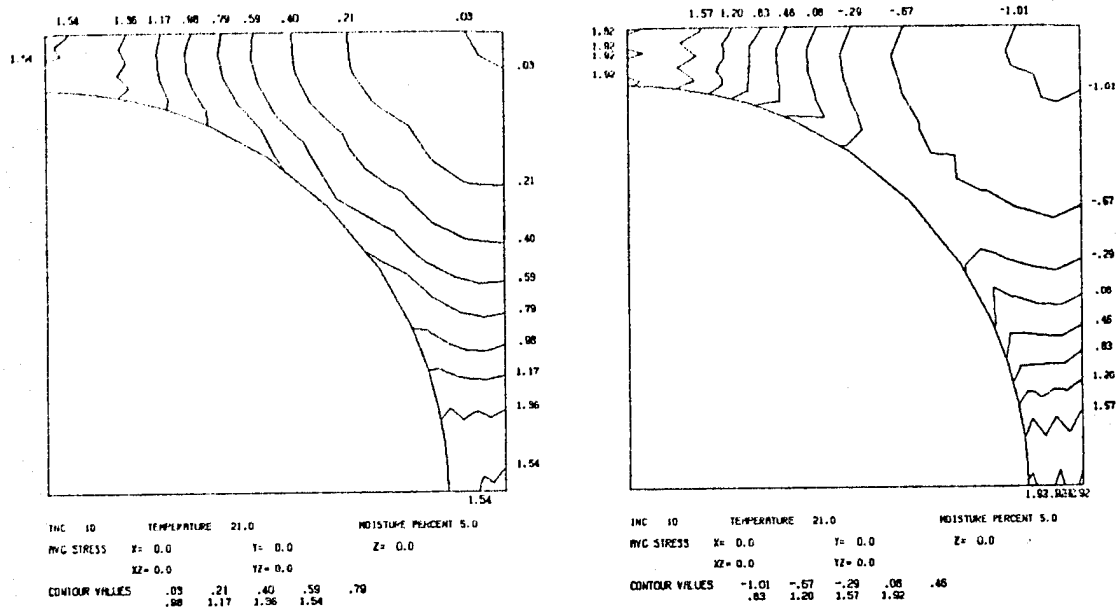
a) Octahedral Shear Stress (ksi)
