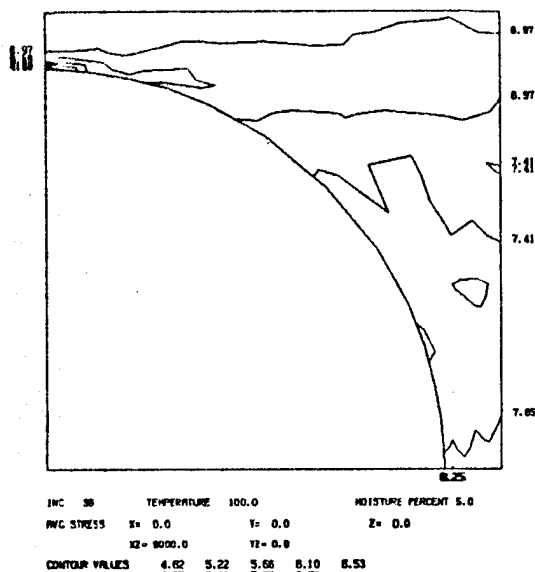
a) Octahedral Shear Stress (ksi)
