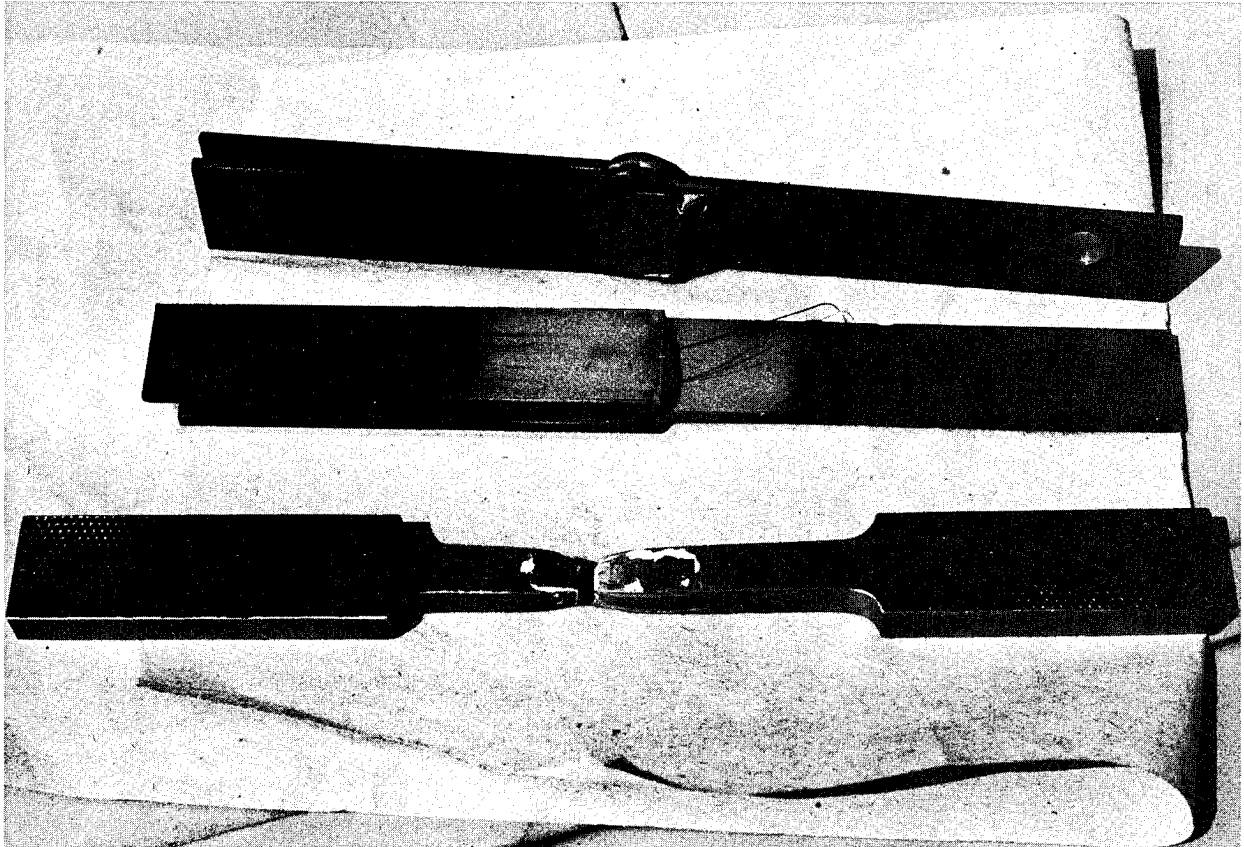
Fig. 1.10 Tensile Specimens
