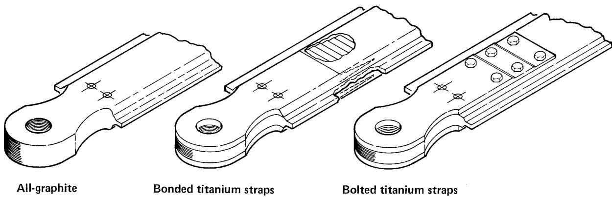
Figure 35. Spar Lug Concepts
