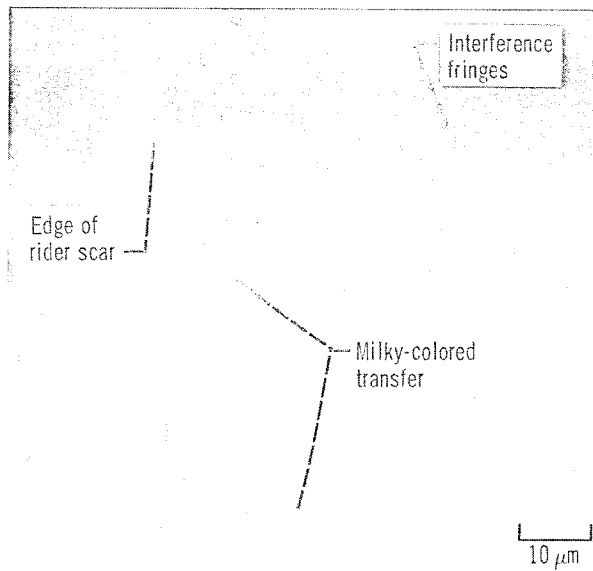
(d) Entrance area (after 8500 kilocycles).
