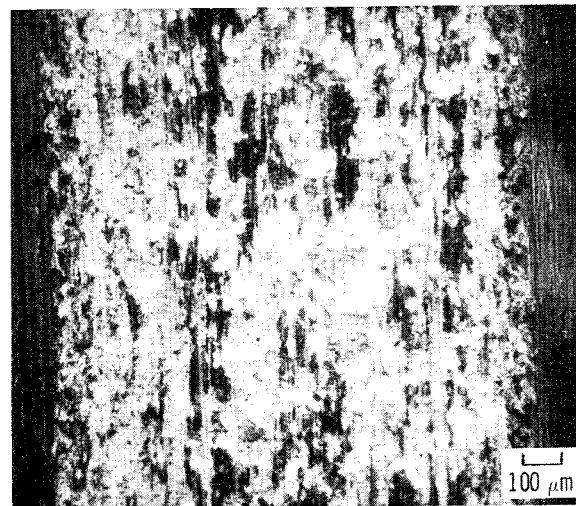
(d) Sliding interval, 8500 kilocycles.
