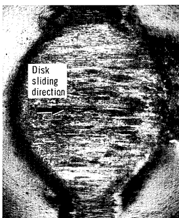
(d) Flat after 1500 kilocycles of sliding.
