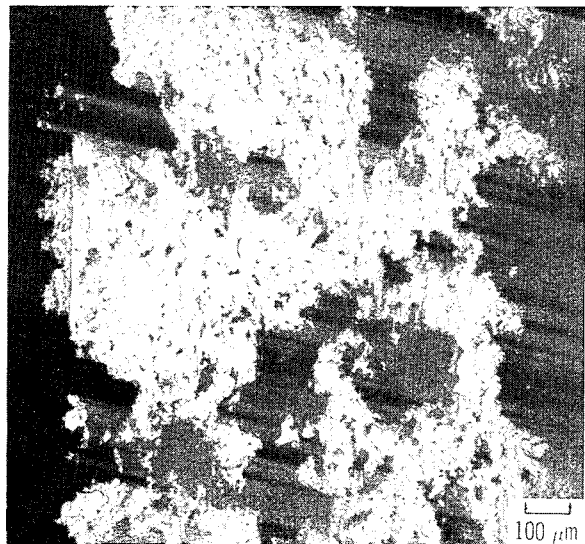
(d) Sliding interval, 250 kilocycles.
