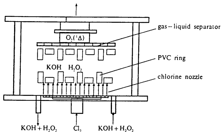
Fig. 2 O 2 ( 1 Δ) generator
