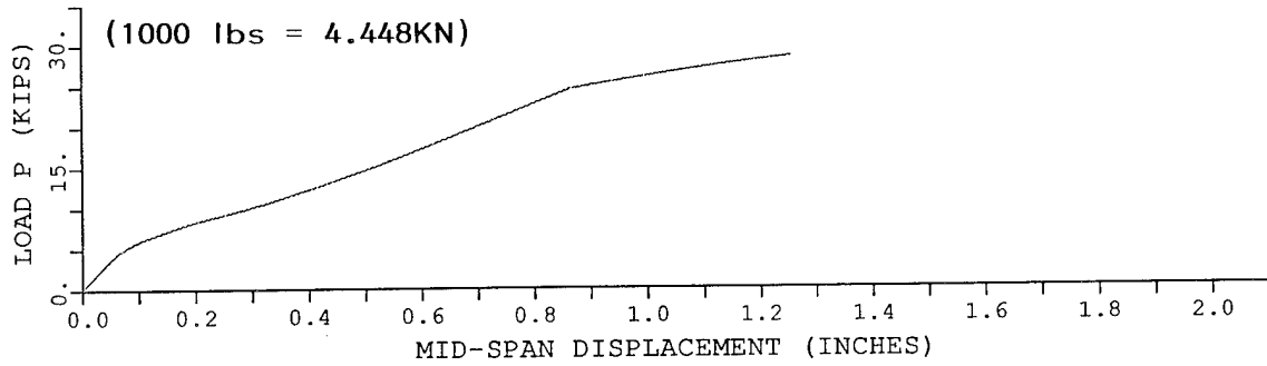
b) load-displacement
