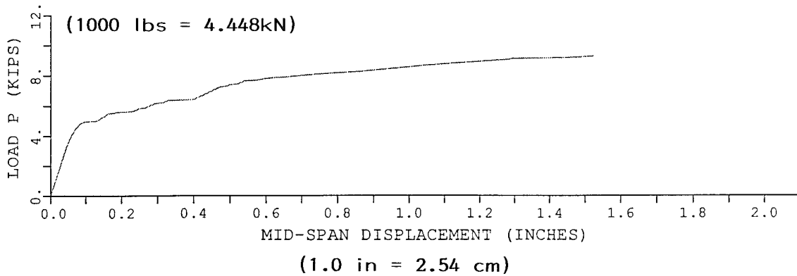
b) load-displacement
