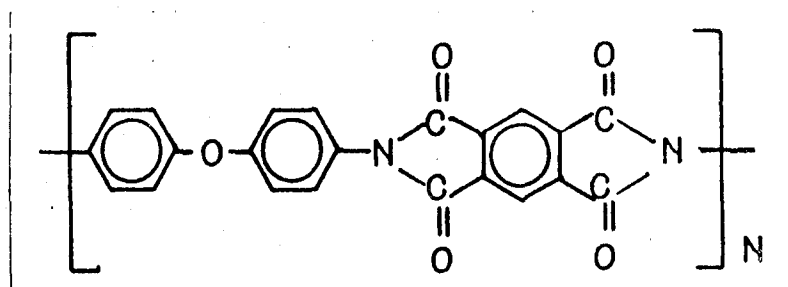
6. Kapton
