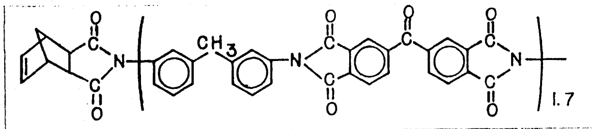
5. LaRC-13
