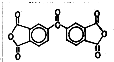
1. BDTA
