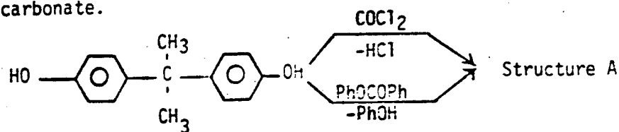
Bisphenol A
