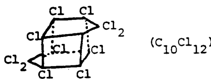
Dechlorane Plus 515
